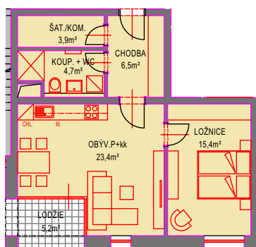
PŮDORYS 1:200
